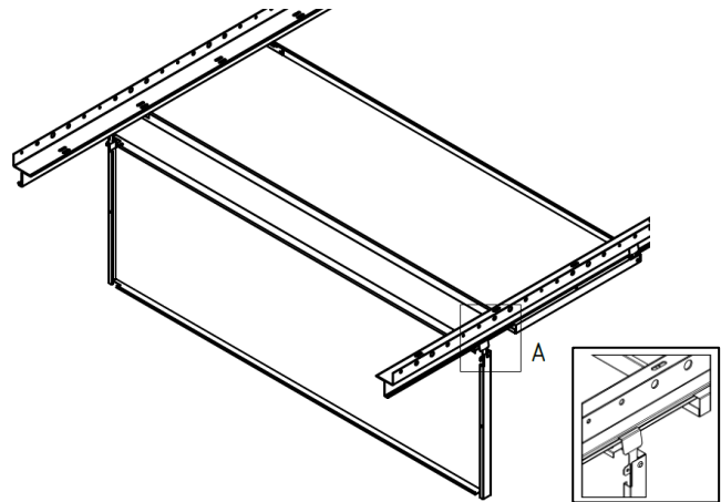
Bild 21 – Beispiel Bandrasterdecke Decklage eingehängt abklappbar
