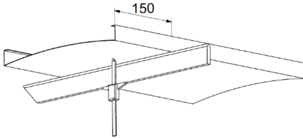
Bild 70 - Prüfung Ebenheit – Wölbung von Paneelen (konkav)
