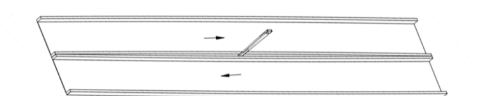
Bild 71 - Prüfung der Säbeligkeit von Paneelen
