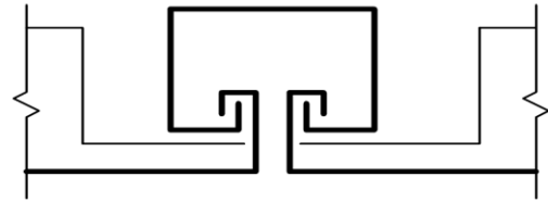
Bild 3 - Beispiel Einhängesystem mit Doppelhängeprofil
