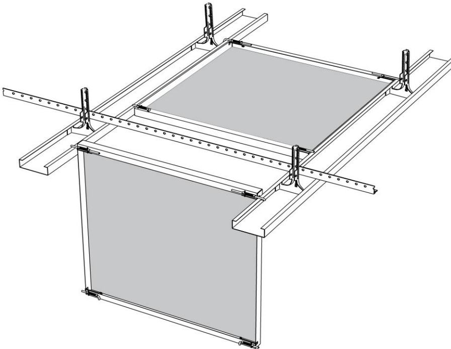
Bild 20 - Beispiel Bandasterdecke – Decklage abklappbar und verschiebbar
