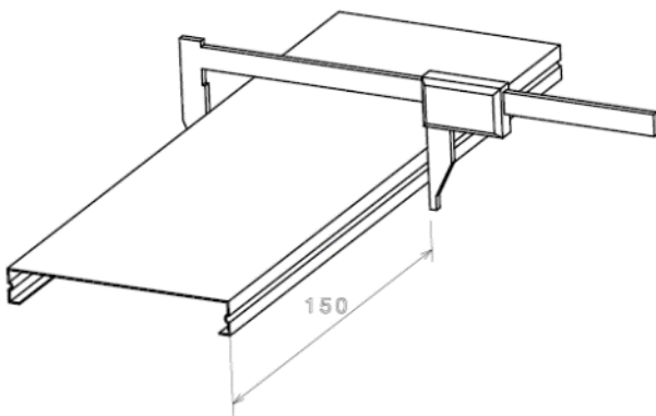
Bild 64 - Prüfung der Paneelbreite
